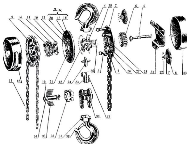
Stirnradflaschenzug
